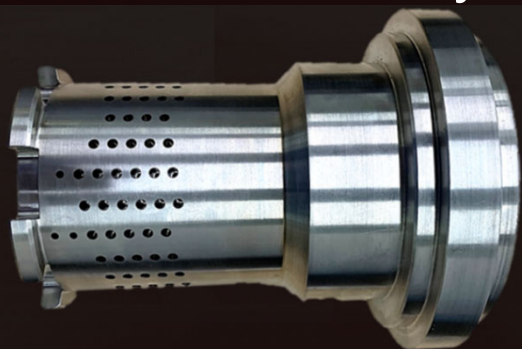
バルブ部品の積層造形品 Laminated model of valve parts 写真提供: 日本ドレッサー(株)
