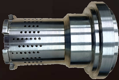
バルブ部品の積層造形品 Laminated model of valve parts
